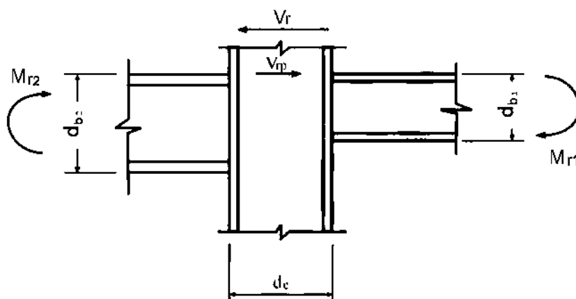
شکل ۱۰-۹-۲-۱۰: برش در چشمه اتصال
