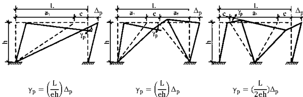
شکل ۳-۱۰-۴-۳-۲: دوران پلاستیک تیر پیوند نسبت به ناحیه خارج از آن ( \gamma_p )
