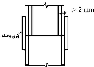
شکل ۲-۱۰-۳-۹-۱۹: نیاز به ورق پرکننده در اتصالات جوشی
