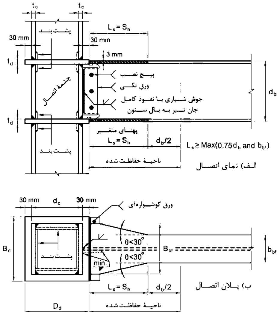
شکل ۱۴-۷-۳-۱۰: اتصال گیردار تیر با بال پهن‌شده و دیافراگم عبوری از ستون (TD-WIDENED)
