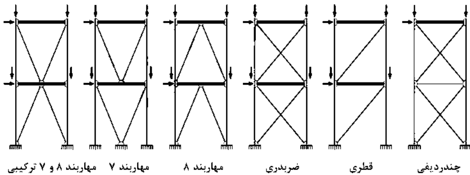
شکل ۱۰-۳-۴-۱-۱: چند نمونه مجاز از پیکربندی مهاربندهای همگرا
