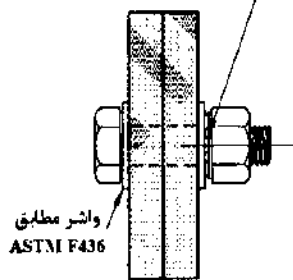
محل اندازه‌گیری فاصله وشر DTI
