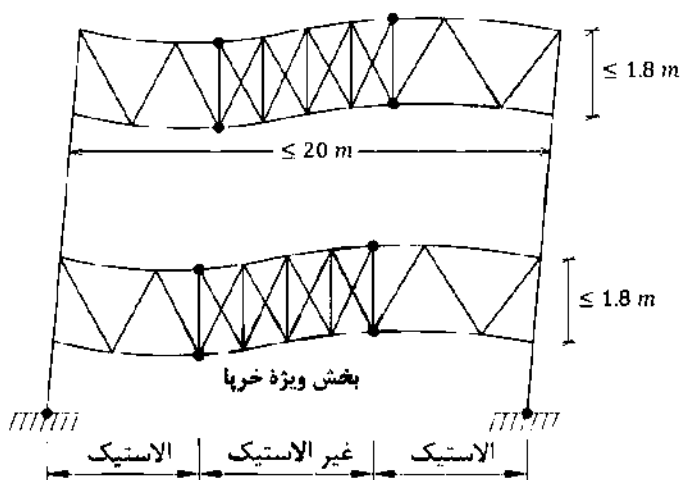
شکل ۱۰-۳-۳-۴: سازوکار تسلیم در بخش ویژه خرپا و رفتار ارتجاعی در سایر بخش‌های خرپا و ستون قاب
