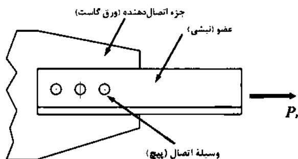
شکل ۱-۹-۲-۱۰: نام‌گذاری قسمت‌های مختلف یک اتصال
