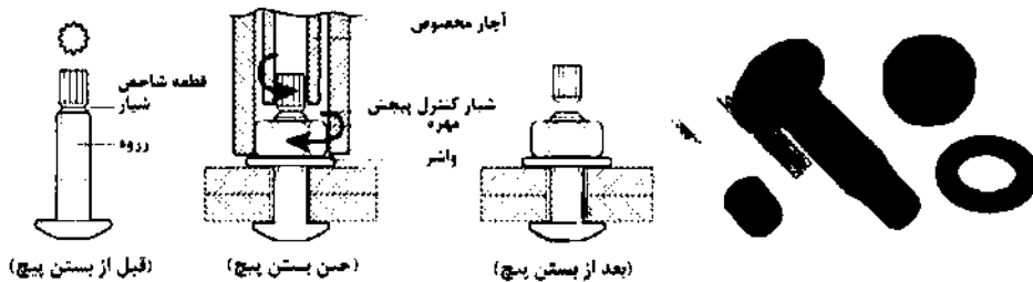
شکل ۵-۴-۱۰: پیچ کشش-کنترل (TC Bolt)
