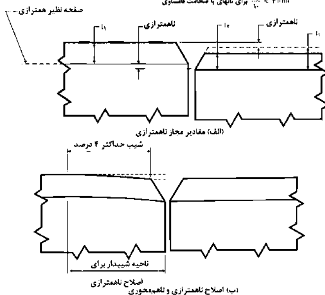
شکل ۱۰-۴-۹: ناهمترای و اصلاح آن
