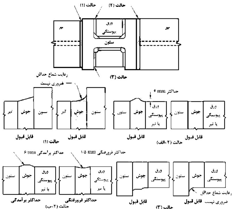
شکل ۴-۲۴: وضعیت‌های قابل قبول برداشتن ورق گوشواره‌ای (ناودان انتهایی جوش)
