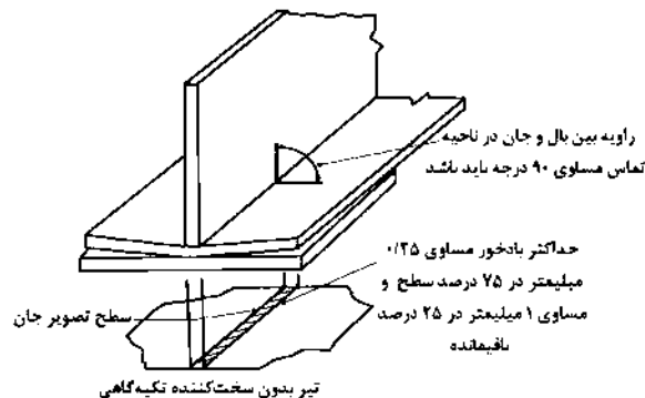
شکل ۴-۱۰-۱۵: رواداری در محل تماس تیر با تکیه‌گاه - تیر بدون سخت‌کننده تکیه‌گاهی
