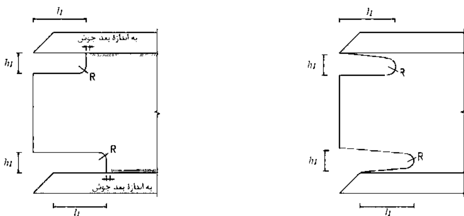
ب) مقاطع ساخته شده از ورق که در آن‌ها ایجاد سوراخ دسترسی قبل از تکمیل جوشکاری بال‌ها به جان صورت می‌گیرد.
