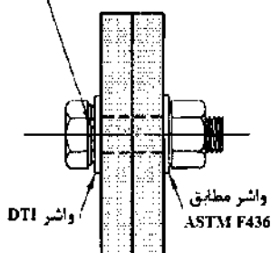
محل اندازه‌گیری فاصله وشر DTI
