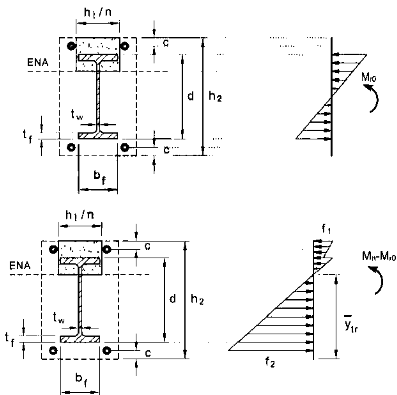
شکل ۲-۱۰-۱۱: مقاومت خمشی مقاطع مختلف محاط در بتن براساس روی هم گذاری تنش های الاستیک
