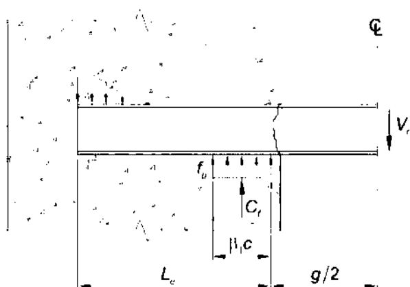
شکل ۱۰-۳-۶-۱: طول آزاد و طول مدفون تیر همبند
