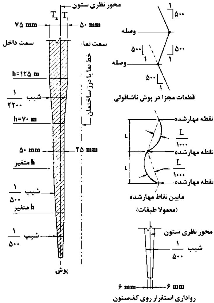
شکل ۱۰-۴-۱۶: پوش ناشاقولی ستون
