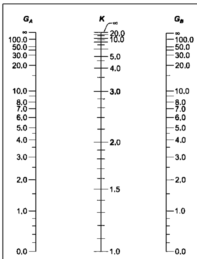
شکل ۱۰-۲-۱: ضریب طول مؤثر (K) اعضای فشاری قاب‌های مهارنشده برحسب G_B و G_A
