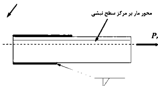
شکل ۱-۹-۲-۱۰: اتصال عضو با مقطع نبشی به ورق اتصال (ورق گاست) از طریق جوش متوازن
