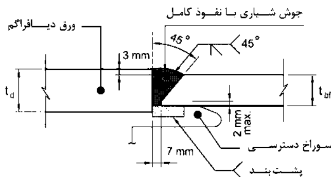
شکل ۱۰-۳-۷: اتصال بال تیر به ورق دیافراگم با استفاده از سوراخ دسترسی و ورق‌های پشت‌بند
