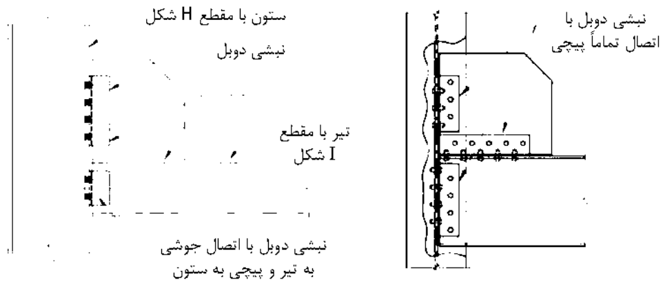
الف) اتصال مفصلی تماماً پیچی به جان ستون ب) اتصال مفصلی جوشی-پیچی به بال ستون
