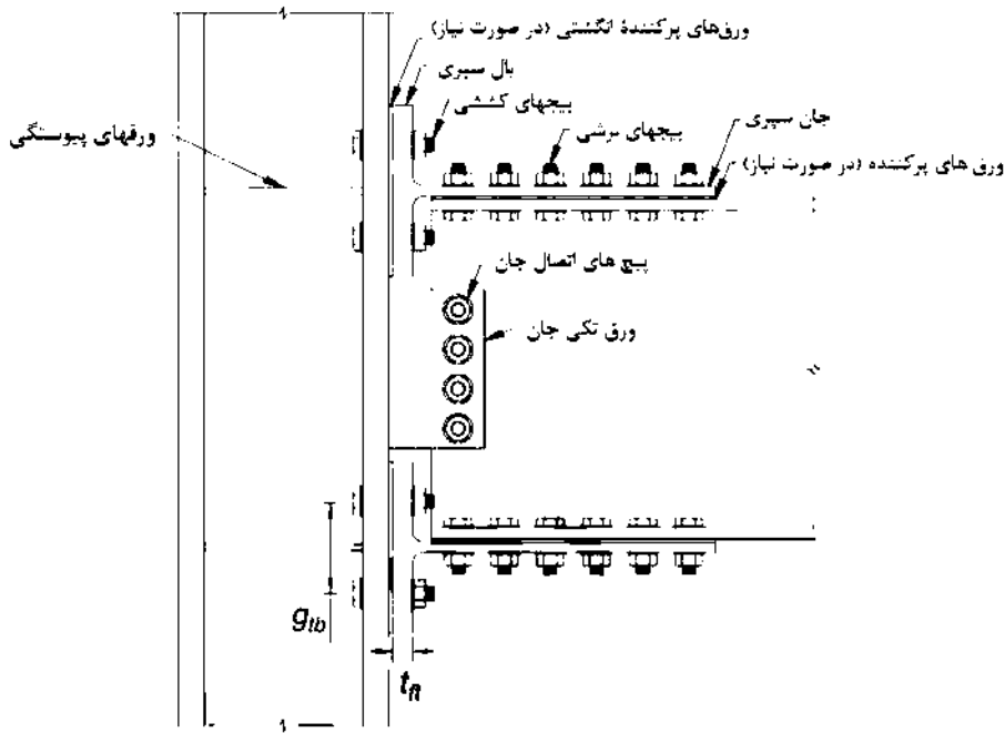
شکل ۸-۷-۳-۱۰: اتصال گیردار پیچی با جفت سپری (DT)
