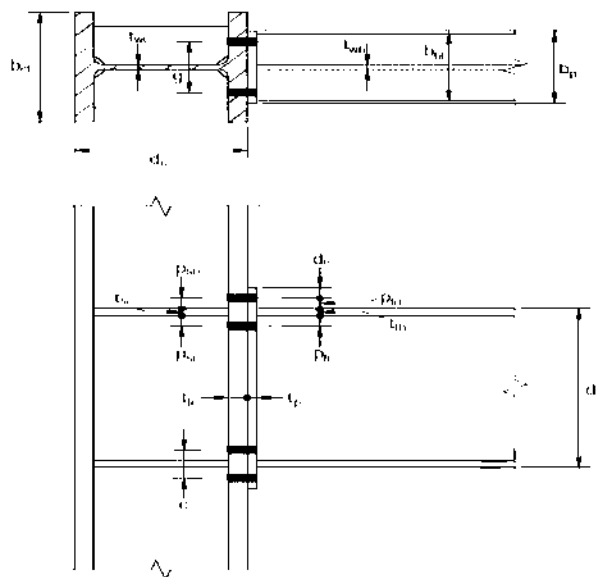
(ت) هندسه اتصال فلنجی چهار پیچی بدون استفاده از ورق لچکی
