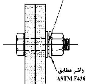
محل اندازه‌گیری فاصله وشر DTI
