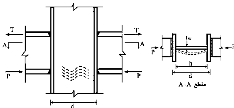
شکل ۱۰-۲-۹-۲۷: کمانش فشاری جان در مقابل یک جفت نیروی متمرکز فشاری
