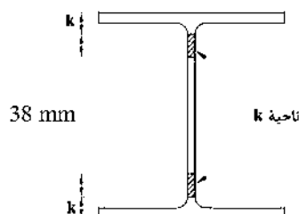
شکل ۴-۱۰: ناحیه k
