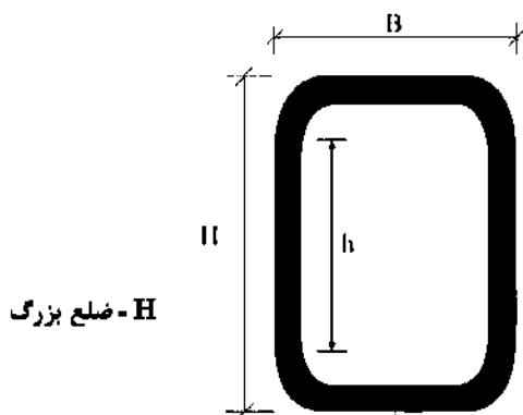
شکل ۱۰-۷-۲-۱: مقطع قوطی شکل
