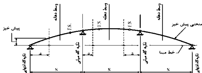
وصله کارگاهی F.S.
