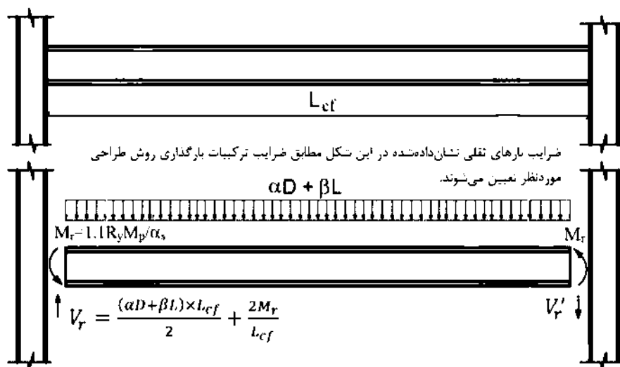
شکل ۱۰-۳-۳-۱: نمودار پیکره آزاد تیرهای باربر لرزه‌ای در قاب‌های خمشی معمولی
