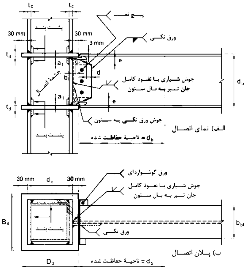
شکل ۱۳-۷-۳-۱۰: اتصال گیردار تقویت نشده جوشی با دیافراگم عبوری از ستون (TD-WUFW)
