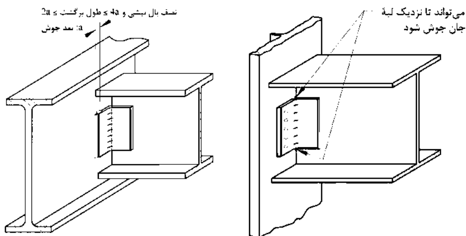
شکل ۱۰-۳-۹-۱۳: اتصالات مفصلی با نبشی جان
