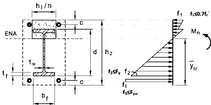
شکل ۱۰-۲-۸: مقاومت خمشی مقاطع مختلف محاط در بتن براساس روی هم گذاری تنش های الاستیک با فرض مقطع تبدیل یافته در حالت استفاده از پایه های موقت
