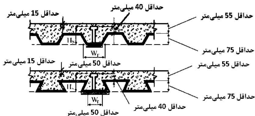
شکل ۱۰-۲-۸-۷: ملاحظات و محدودیت‌های عرشه فولادی برای حالت یک گل‌میخ در پهنای
