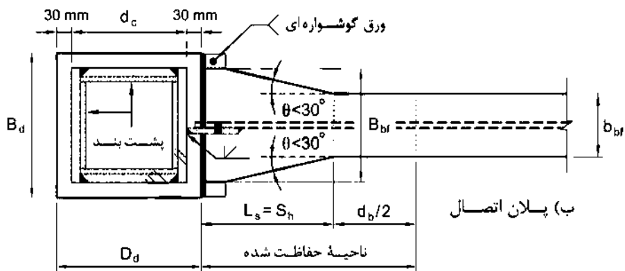
شکل ۳-۱۰-۷-۱۶: اتصال گیردار تیر با بال پهن شده و دیافراگم عبوری از ستون (TD-WIDENED) در قاب‌های خمشی متوسط
