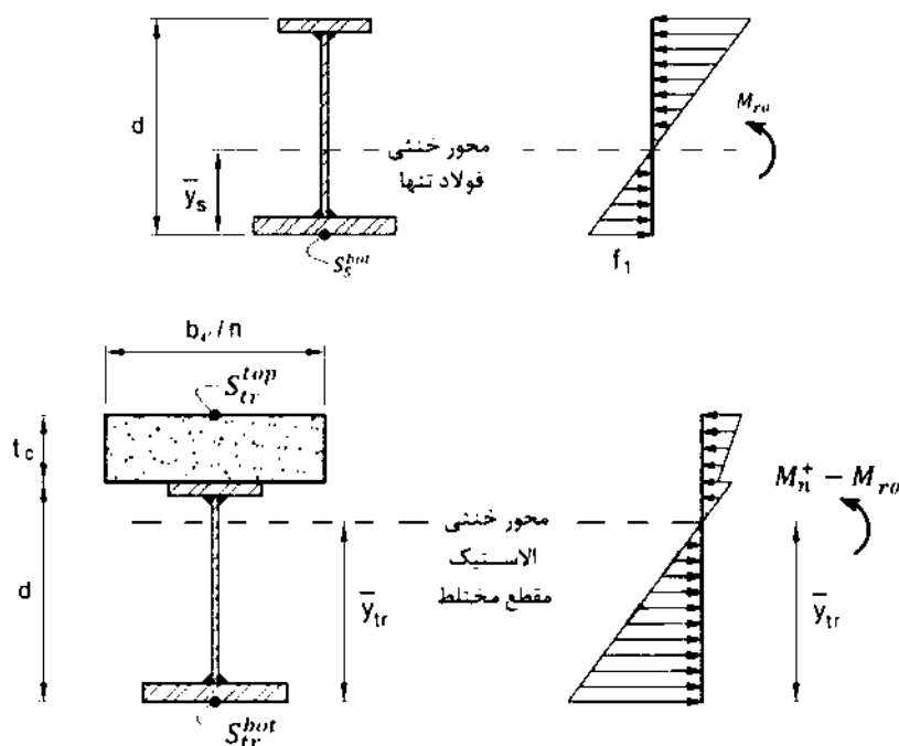
شکل ۵-۸-۱۰: توزیع الاستیک تنش در مقطع مختلف تبدیل یافته در صورت عدم استفاده از پایه‌های موقت
