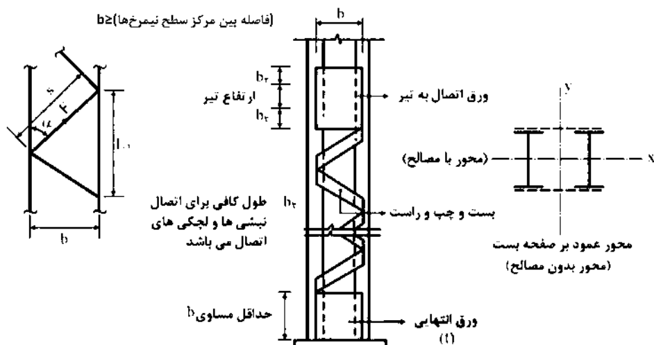
شکل ۲-۱۰-۳: عضو فشاری ساخته شده (مرکب) با بست‌های مورب
