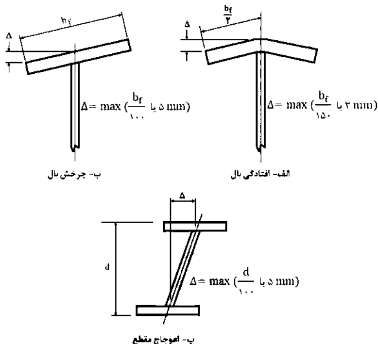
شکل ۱۳-۴-۱۰: رواداری های انحراف بال
