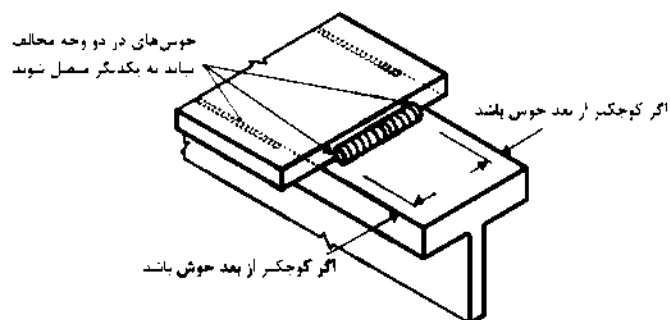
شکل ۱۰-۳-۹-۱۴: جوش‌های گوشه در دو وجه مخالف یک صفحه مشترک
