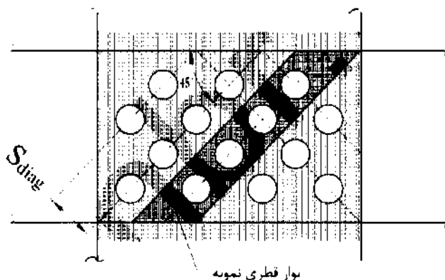
شکل ۱۰-۳-۴-۵: آرایش سوراخ‌ها در دیوارهای برشی فولادی ویژه سوراخ‌دار
