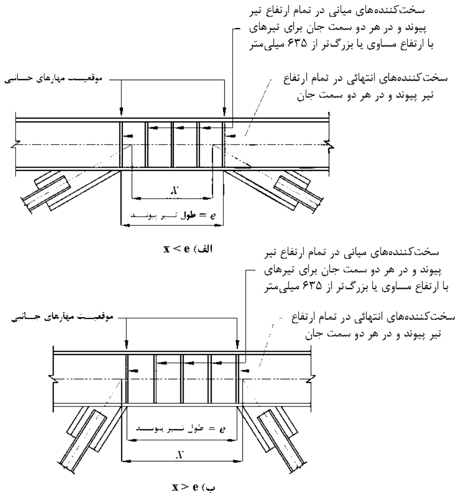
شکل ۱۰-۳-۴-۳: تیر پیوند با مقطع I شکل و سخت‌کننده‌های موردنیاز
