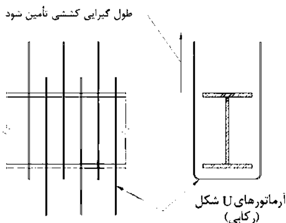
شکل ۱۰-۳-۶-۳: استفاده از آرماتورهای U شکل به عنوان میلگردهای انتقال
