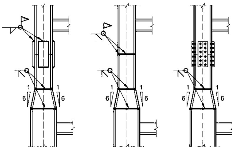
شکل ۱۰-۳-۴۰: جزئیات پیشنهادی وصله ستون‌ها در محل تغییر قابل ملاحظه مقطع
