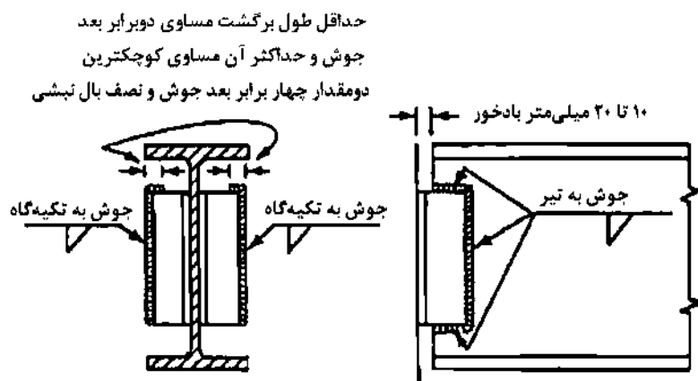
شکل ۱۰-۳-۵: جزئیات اتصال جوشی با استفاده از نبشی جفت در جان
