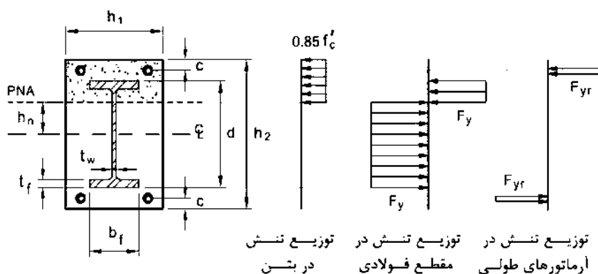
شکل ۲-۱۰-۸: مقاومت خمشی مقاطع مختلف محاط در بتن براساس روش توزیع تنش پلاستیک
