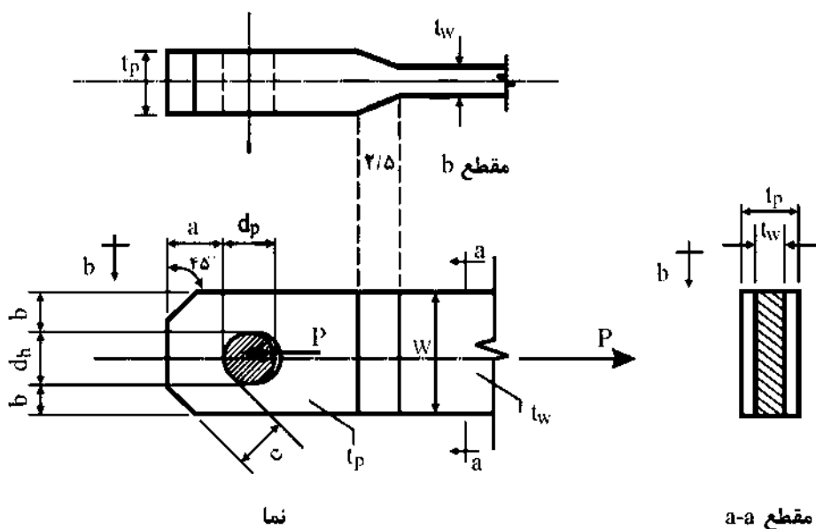
شکل ۱۰-۴-۱: محدودیت‌های ابعادی تسمه لولا شده با خار مغزی
