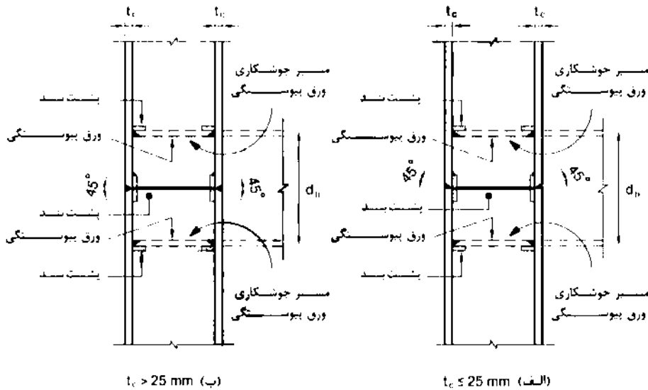
شکل ۳-۲-۳-۱۰: گزینه دیگر موقعیت وصله کارخانه‌ای ستون‌ها
