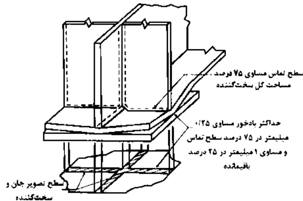
شکل ۴-۱۰-۱۴: رواداری در محل تماس تیر با تکیه‌گاه - تیر با سخت‌کننده تکیه‌گاهی
