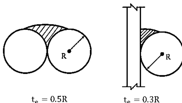
شکل ۸-۹-۲-۱۰: ضخامت مؤثر جوش‌های شیار لب‌گرد
