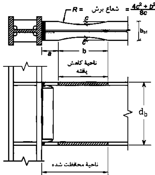
شکل ۳-۱۰-۲-۷-۳: اتصال گیردار تیر با مقطع کاهش یافته (RBS)
