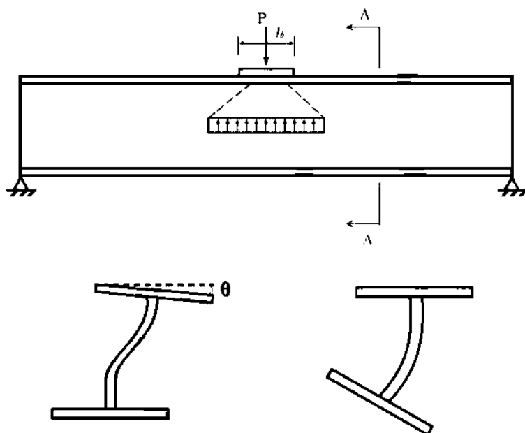
(ب) بال فشاری در مقابل دوران زاویه‌ای نگهداری نشده است. (مقطع A-A)
