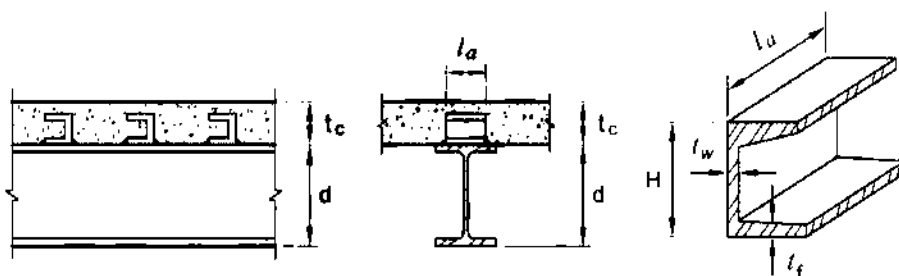
شکل ۱۰-۲-۸-۱۷: برشگیرهای از نوع ناودانی
