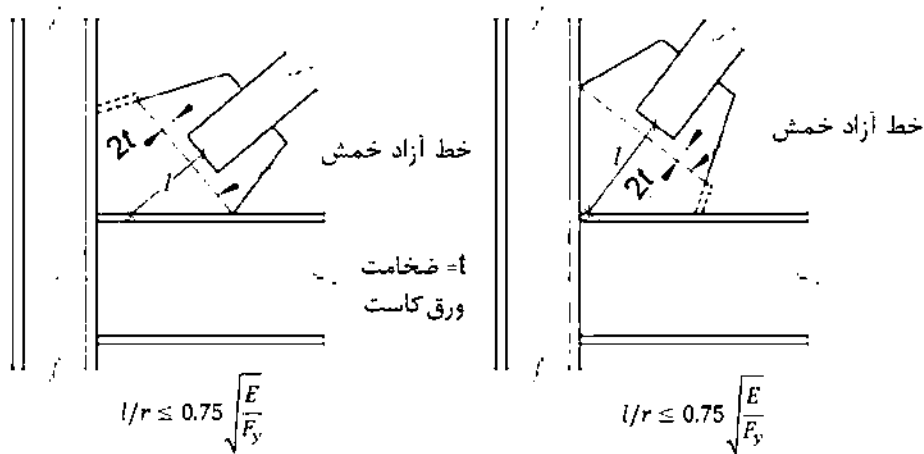
شکل ۳-۱۰-۴-۳: سازگاری ورق اتصال (ورق گاست) با کمانش خارج از صفحه عضو مهاربندی
