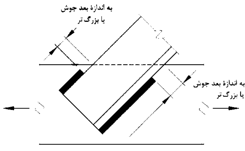
شکل ۱۰-۲-۹-۱۱: جوش گوشه در انتهای اعضای محوری
