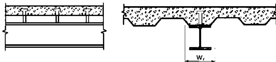
شکل ۲-۱۰-۹-۸: عرشه فولادی که کنگره‌های آن موازی با محور طولی تیر است
