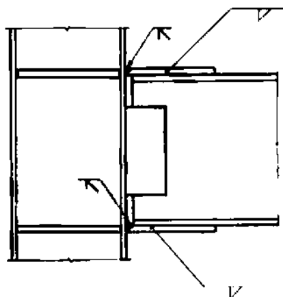
شکل ۱۰-۳-۶: جزئیات یک نمونه از اتصال گیردار تیر به ستون با ورق جوش شده
