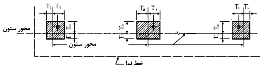
شکل ۱۰-۴-۱۸: تاراستایی ستون‌های داخلی
