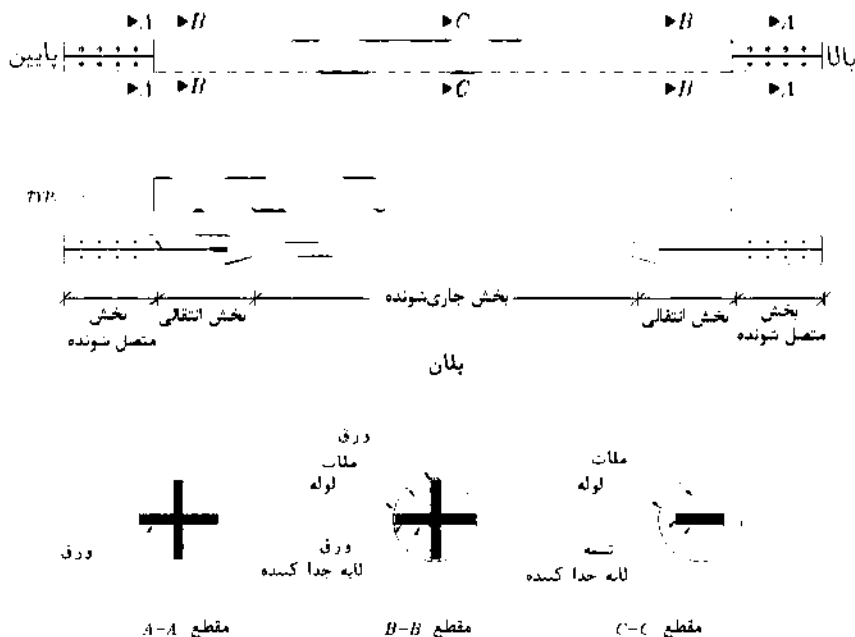
شکل ۳-۱۰-۴-۱: نمونه‌ای از اجزای یک مهاربند کمانش تاب
