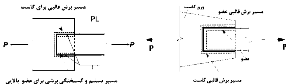
(ب) برخی دیگر از حالت‌های گسیختگی برش قالبی
