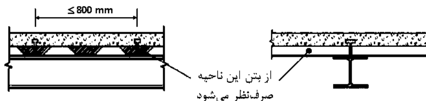
شکل ۲-۱۰-۸-۸: عرشه فولادی که کنگره‌های آن عمود بر محور طولی تیر است
