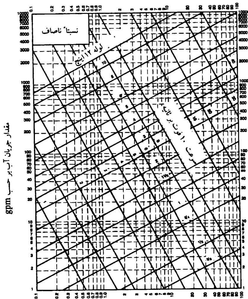
افت فشار آب بر حسب فوت در ۱۰۰ فوت طول
